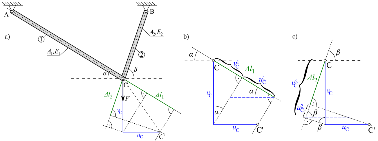
Rys. 7: Układ dwóch prętów; statycznie wyznaczalny
