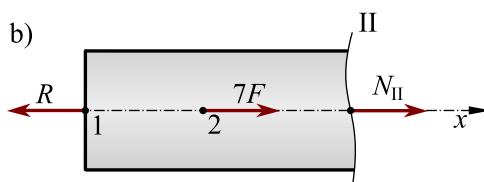
Rys. 4: Pręt stopniowany obciążony kilkoma siłami statycznie wyznaczalny
