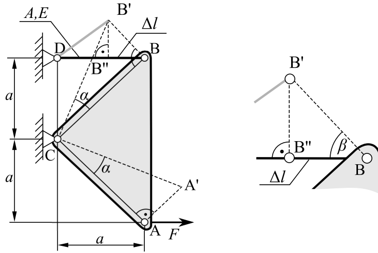
Rys. 9: Analiza przemieszczeń punktów układu
